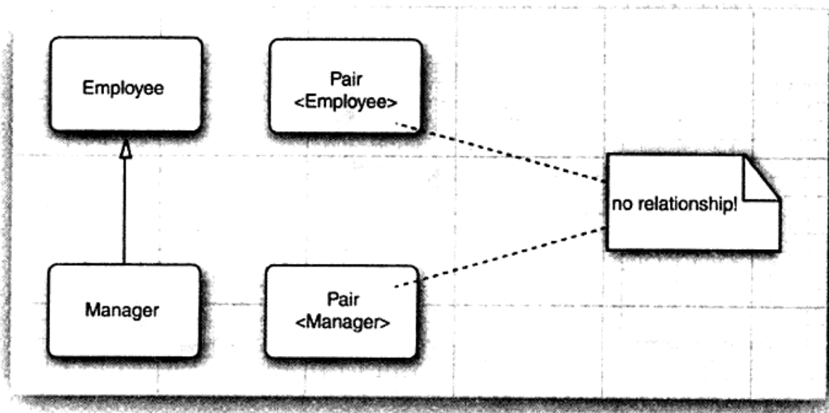
图12-1 pair类之间没有继承关系
