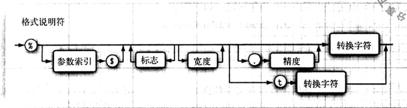
图3-6 格式说明符语法
