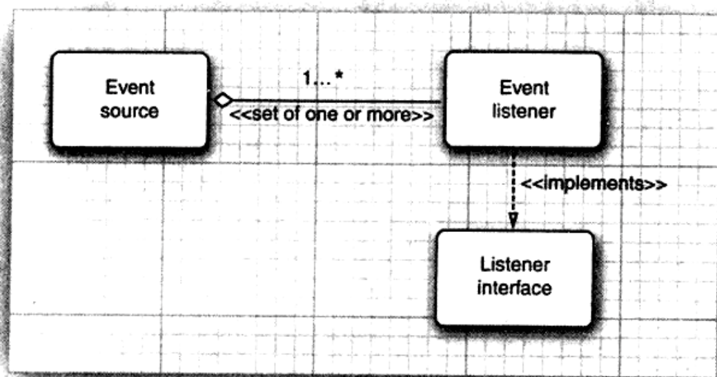
图8-1 事件源和监听器之间的关系
