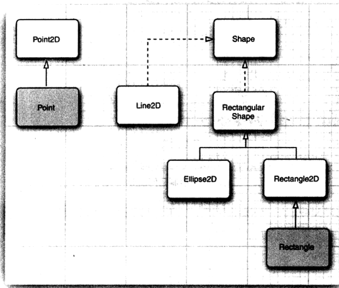
图7-10 图形类之间的关系
