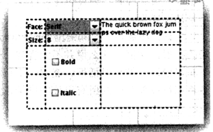
图9-30 设计中使用的对话框网格
