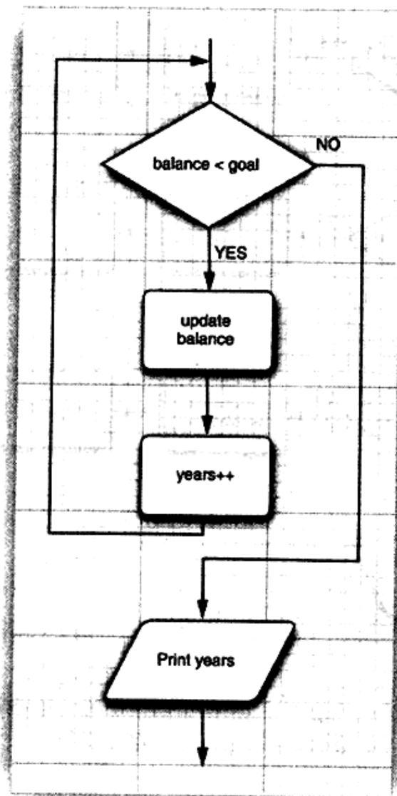
图3-10 while语句的流程图
