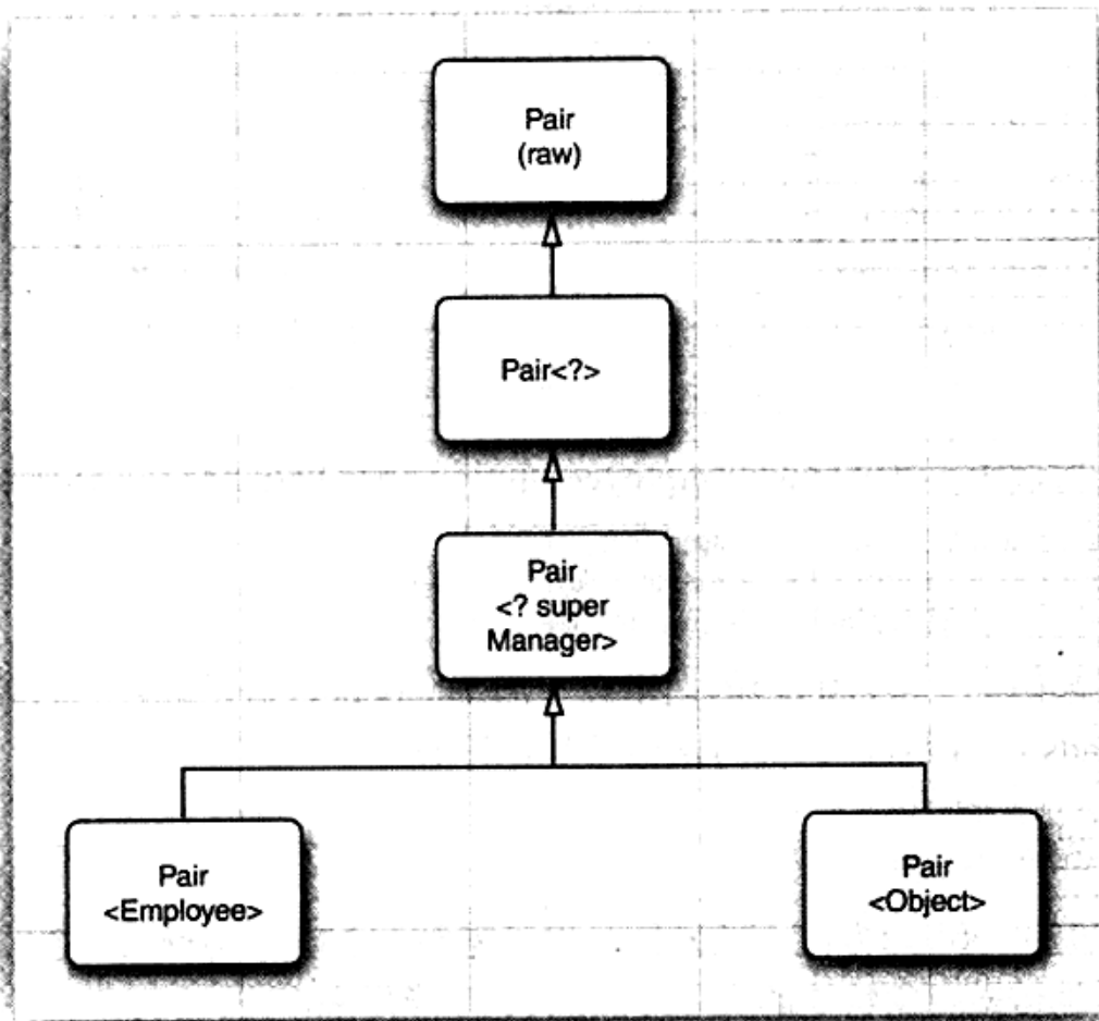
图12-4 带有超类型边界的通配符
