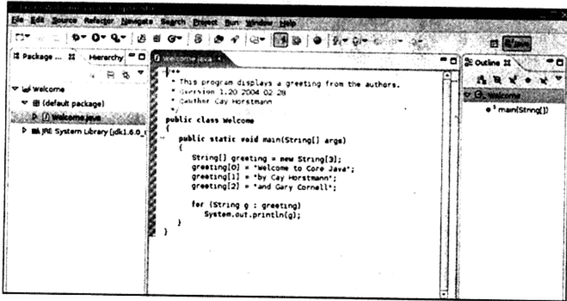
图2-6 使用Eclipse编辑源文件
