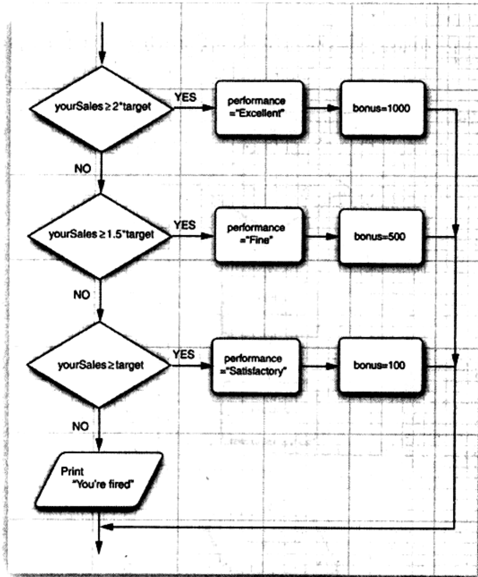
图3-9 if/else if (多分支) 的流程图
