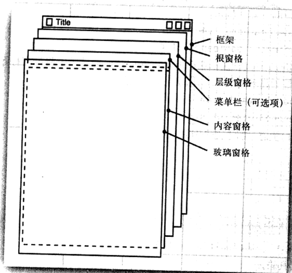
图7-7 JFrame的内部结构
