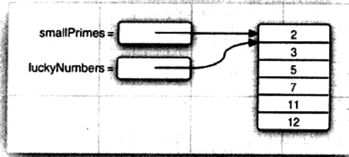
图3-14 拷贝一个数组变量
