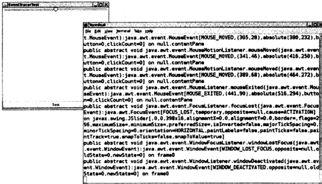
图11-5 The Eventtracer 类的运行结果
