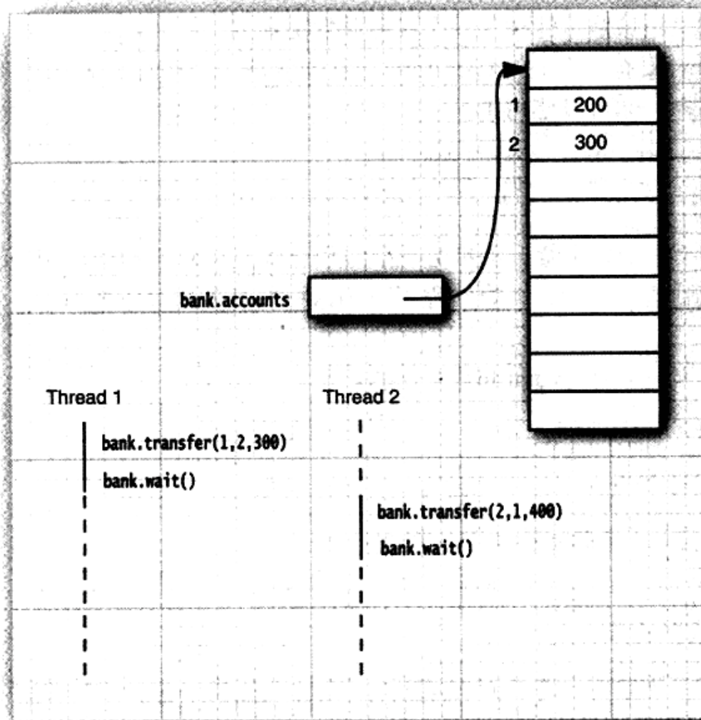
图14-6 发生死锁的情况
