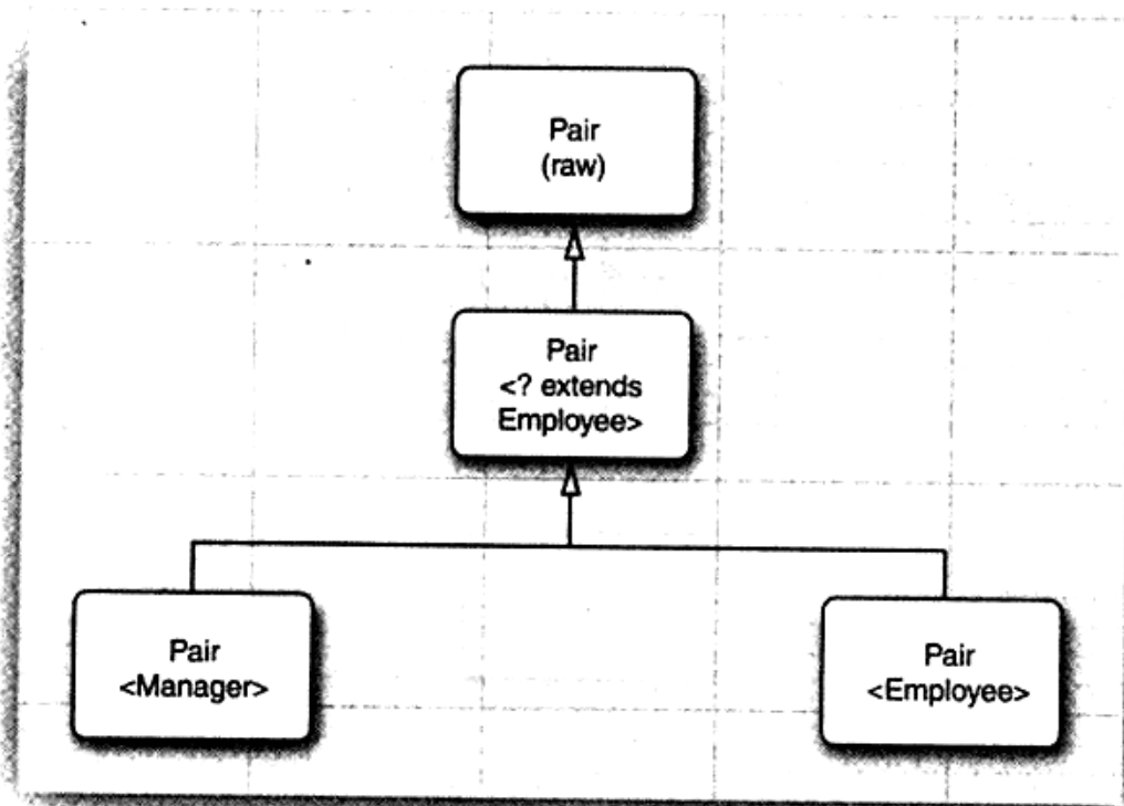
图12-3 使用通配符的子类型的联系
