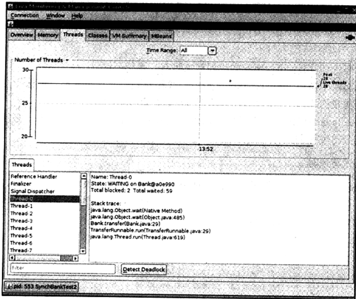
图14-7 jconsole中的线程面板
