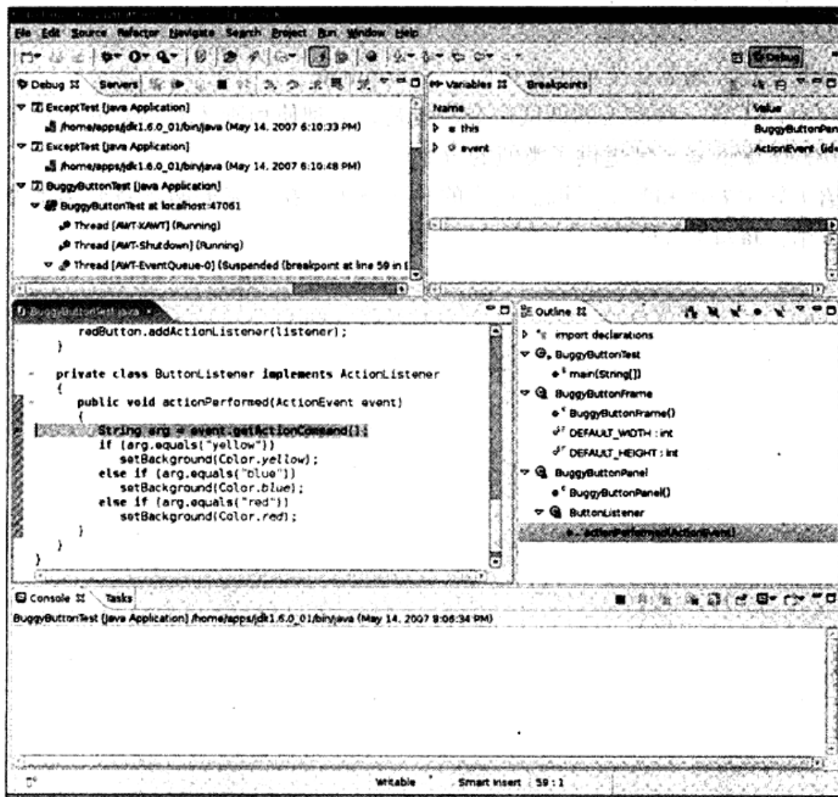
图11-7 停止在断点处
