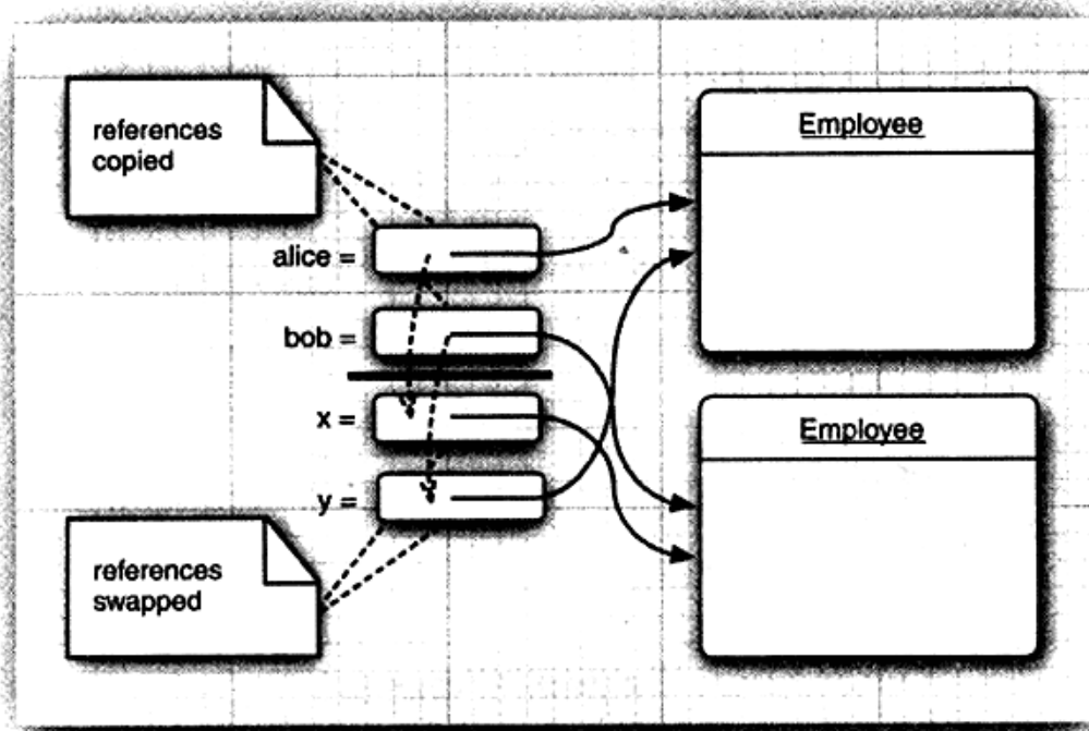
图4-8 交换对象参数的结果没有被保下来
