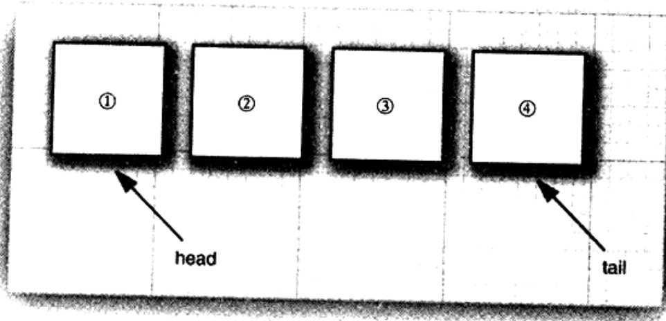
图13-1 队列
