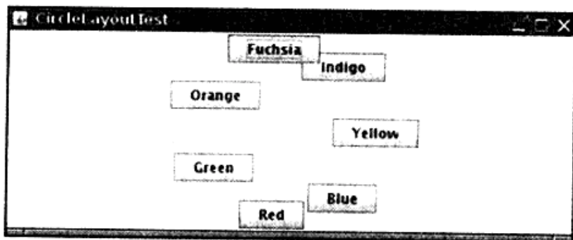
图9-34 圆形布局
