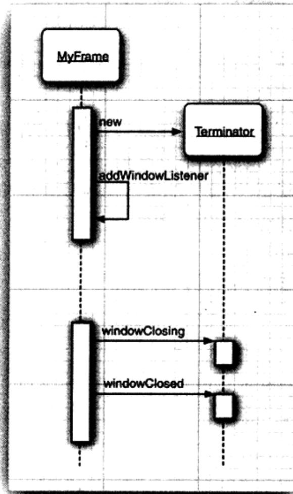
图8-5 窗口监听器
