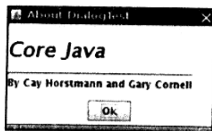
图9-38 About对话框
