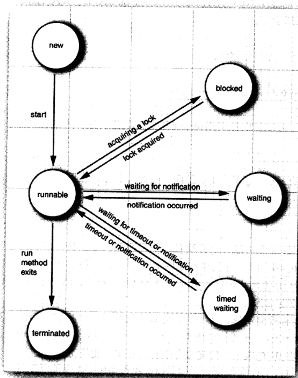
图14-3 线程状态
