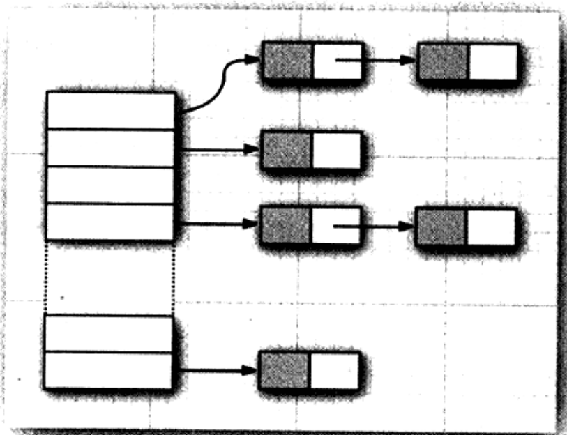
图13-8 散列表
