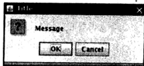
图9-36 选项对话框
