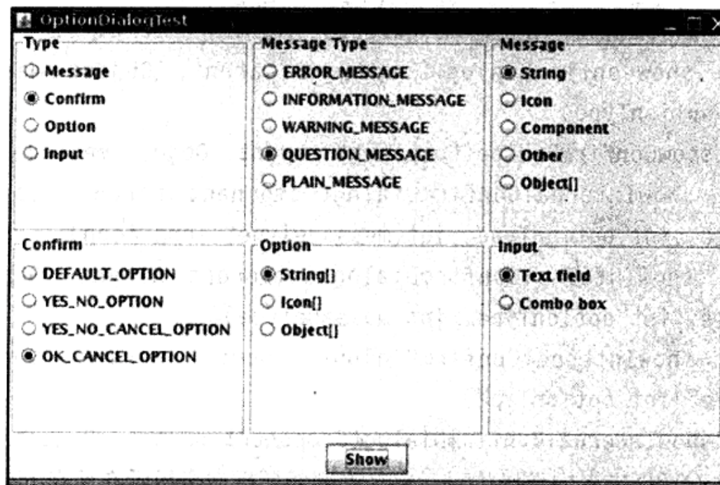
图9-37 OptionDialogTest程序
