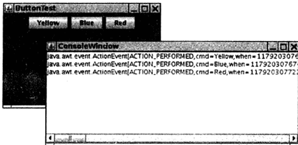
图11-4 控制台窗口
