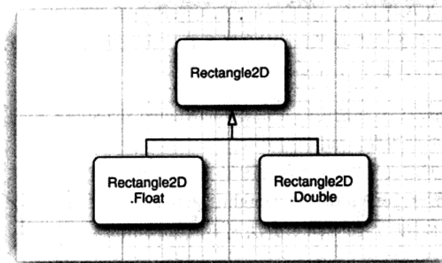
图7-8 2D矩形类
