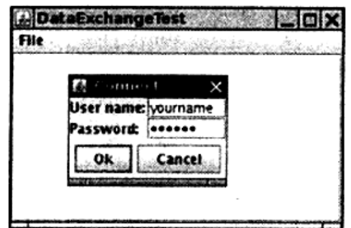
图9-39 密码对话框
