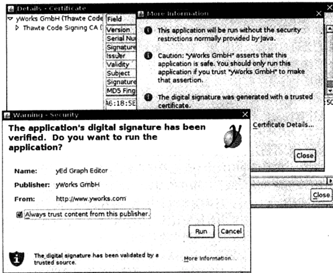
图10-6 安全认证书
