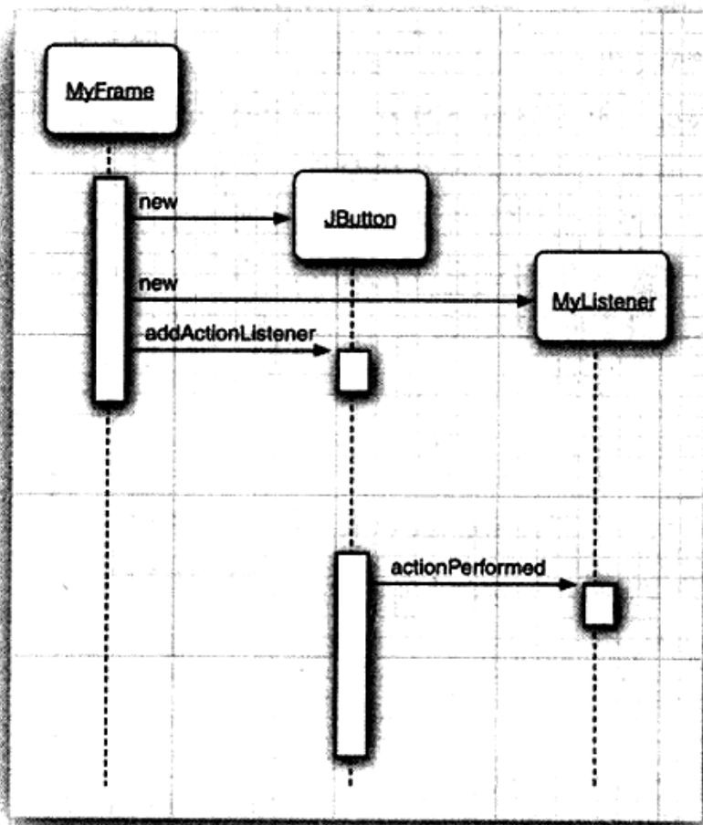
图8-2 事件通告
