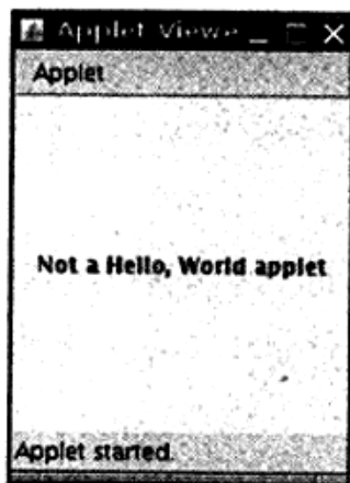
图10-15 Applet程序
