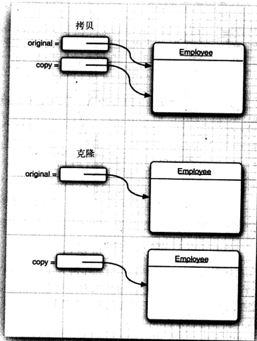
图6-1 拷贝与克隆
