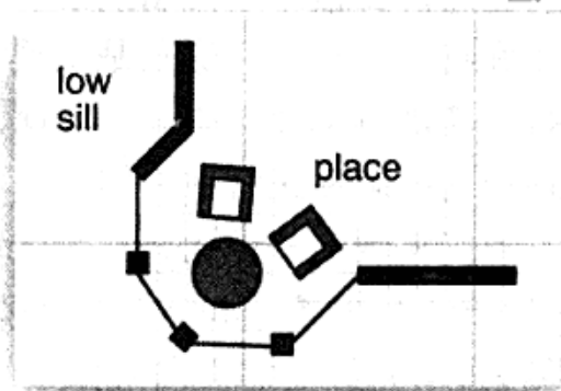
图9-1 窗户位置
