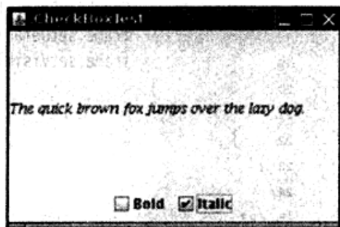
图9-14 复选框
