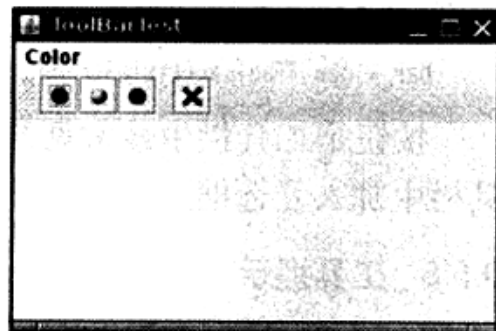
图9-24 工具栏
