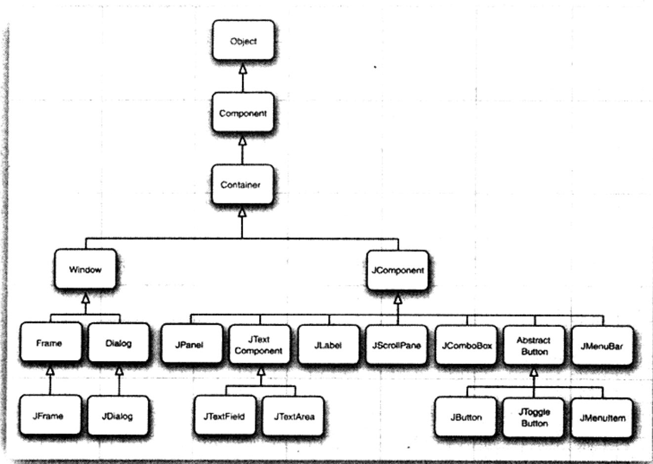
图9-8 Component的类层次结构
