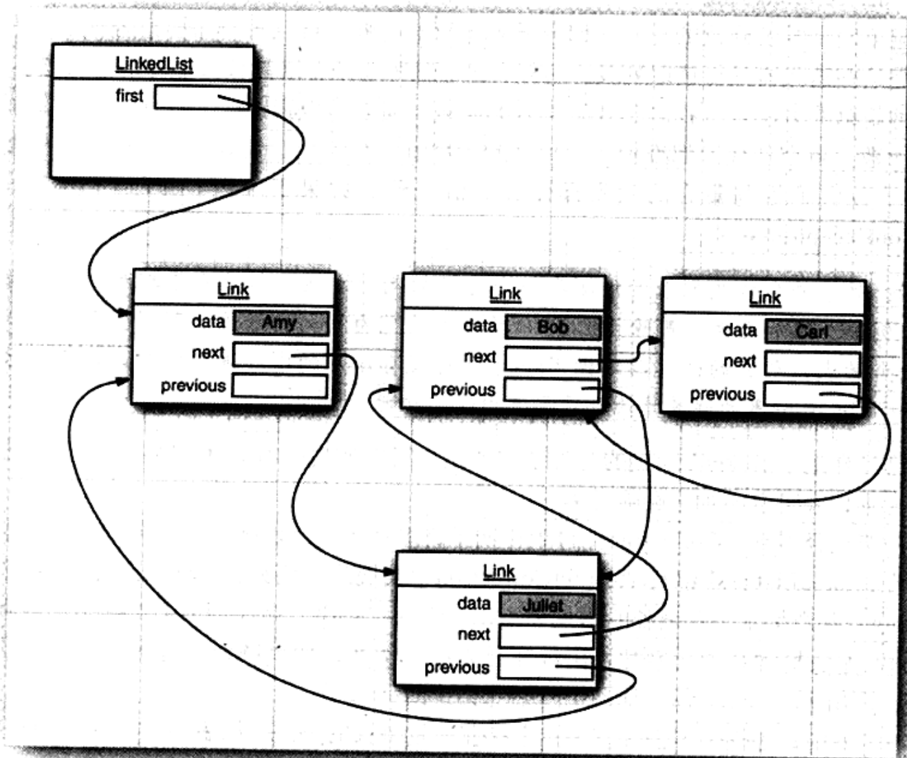
图13-7 将一个元素添加到链表中
