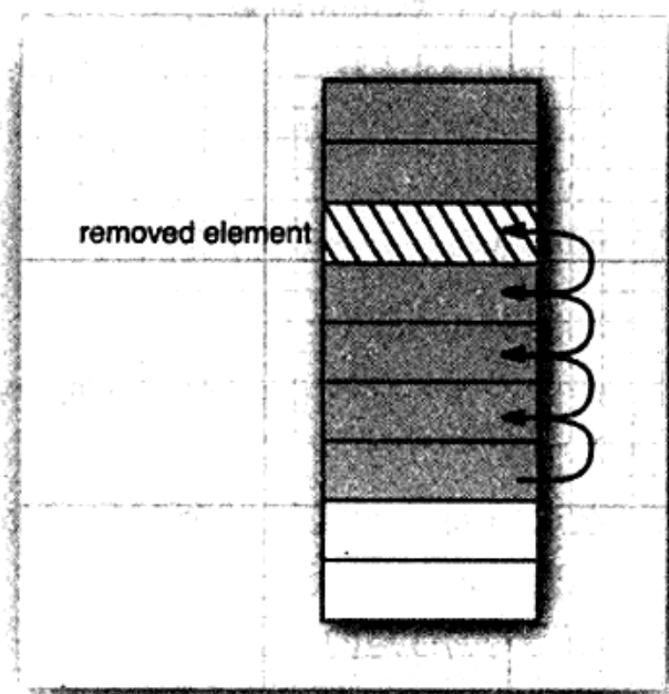
图13-4 从数组中删除一个元素
