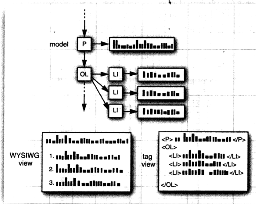
图9-3 同一模型的两个不同视图
