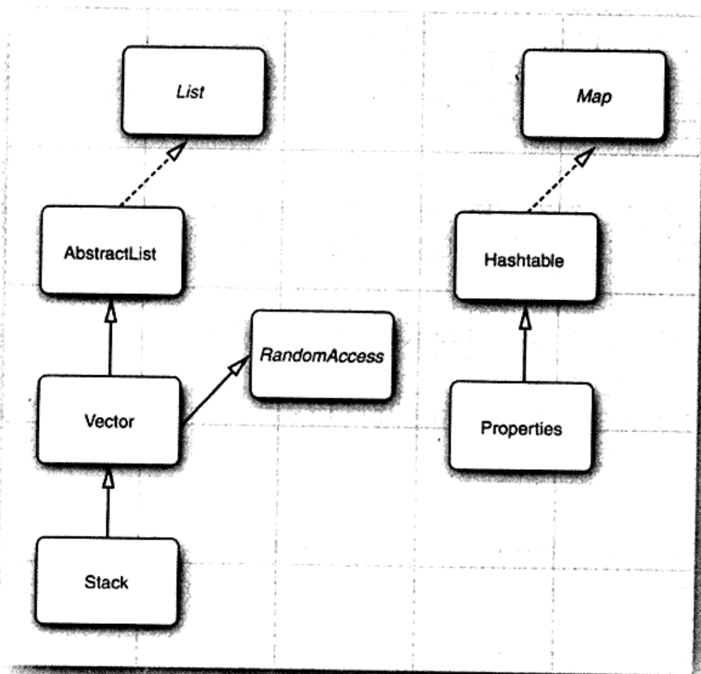
图13-12 集合框架中的遗留类
