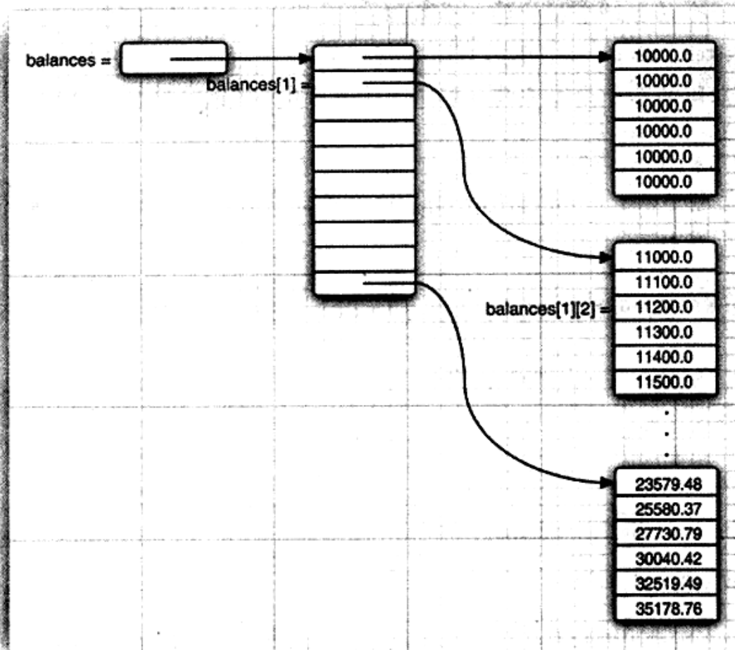
图3-16 一个二维数组
