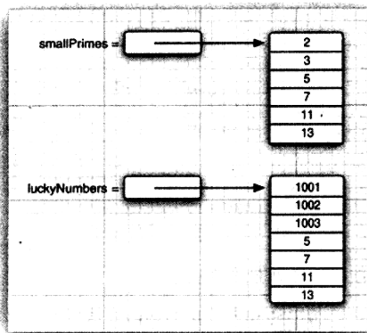
图3-15 数组之间拷贝元素值
