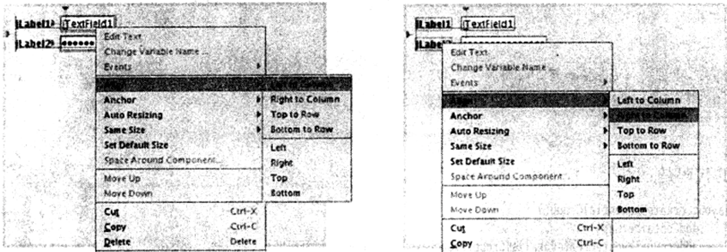
图9-32 在Matisse中对齐标签和文本域
