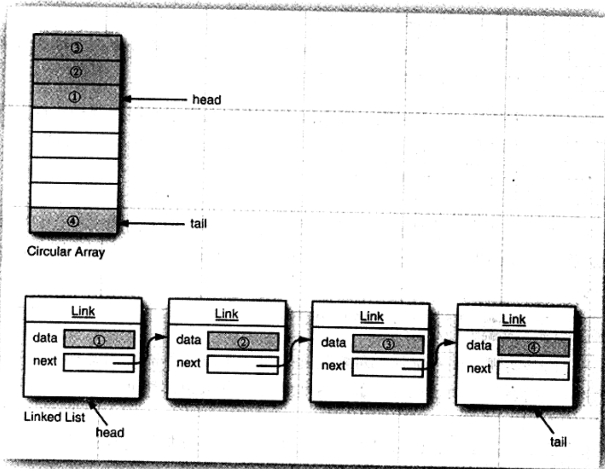
图13-2 队列的实现
