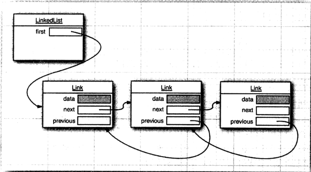
图13-5 双向链表
