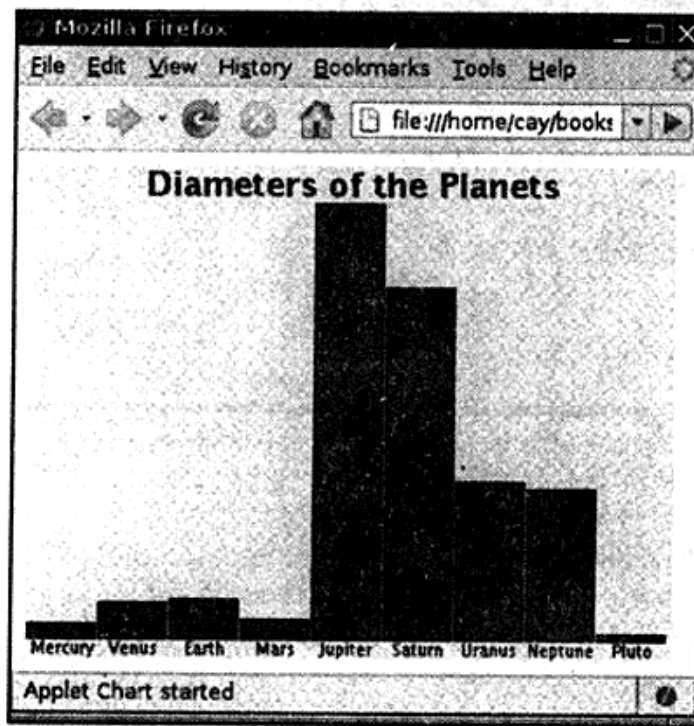
图10-14 图表applet
