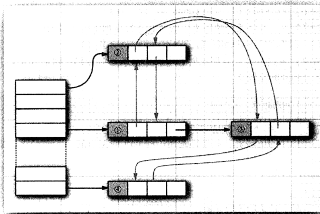
图13-9 链接散列表
