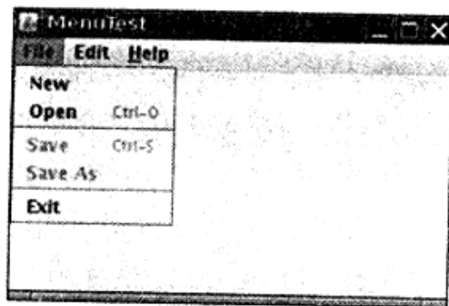
图9-22 加速器
