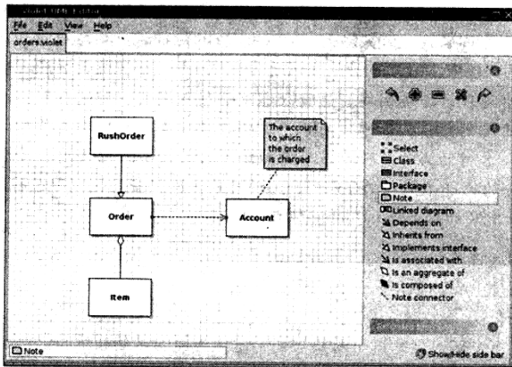
图4-2 类的示意图
