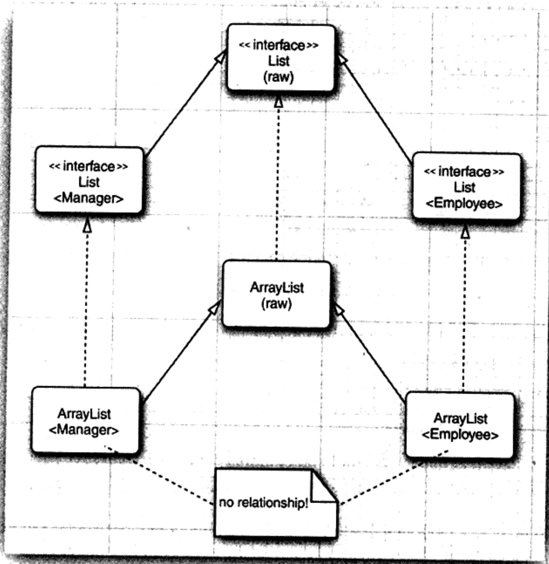
图12-2 泛型列表类型中子类型间的联系
