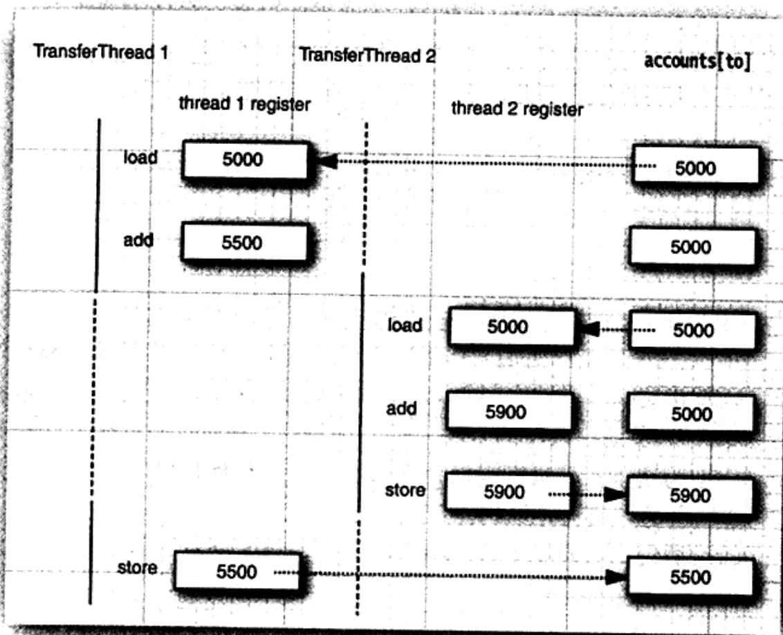
图14-4 同时被两个线程访问
