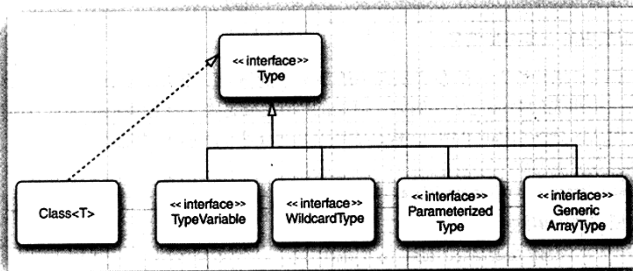
图12-5 Type类和它的后代
