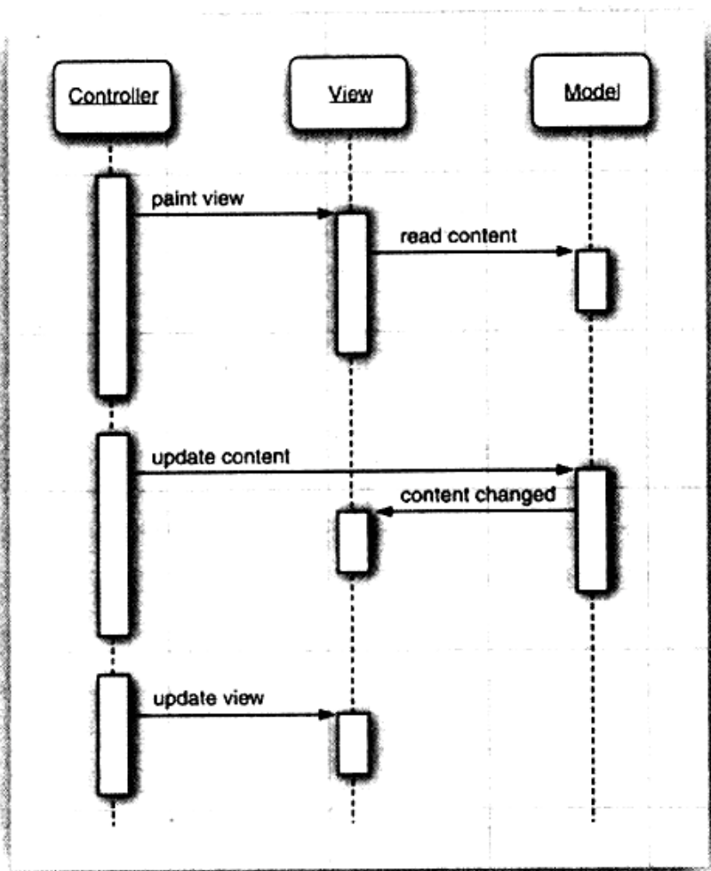
图9-4 给出了模型、视图、控制器对象之间的交互。
