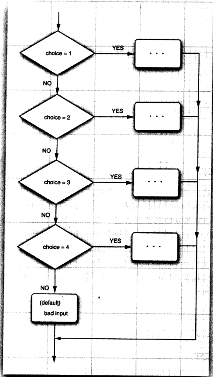
图3-13 switch语句的流程图
