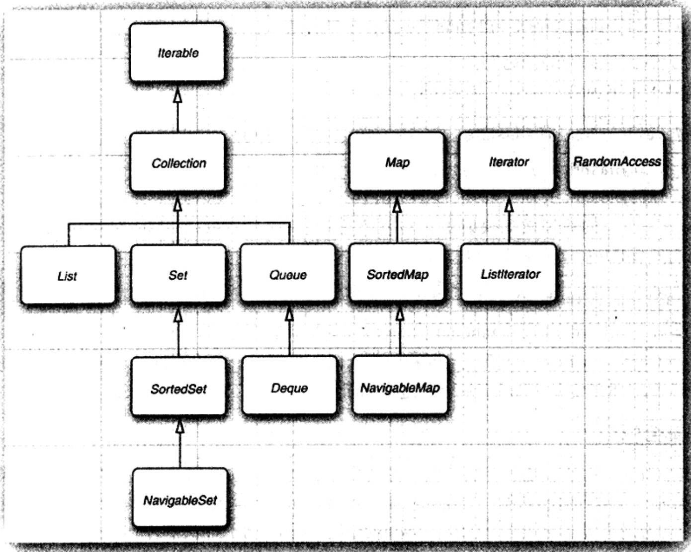
图13-10 集合框架的接口
