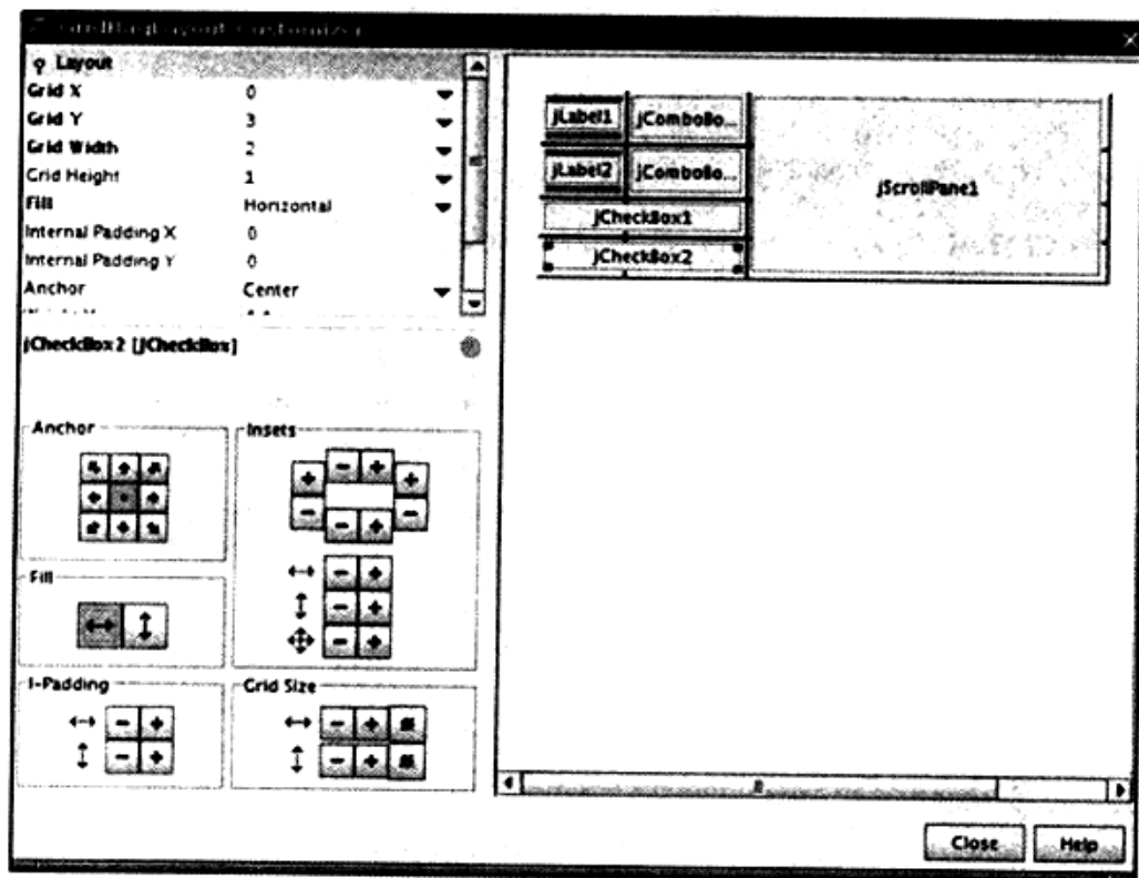
图9-31 在NetBeans中指定网格组的约束
