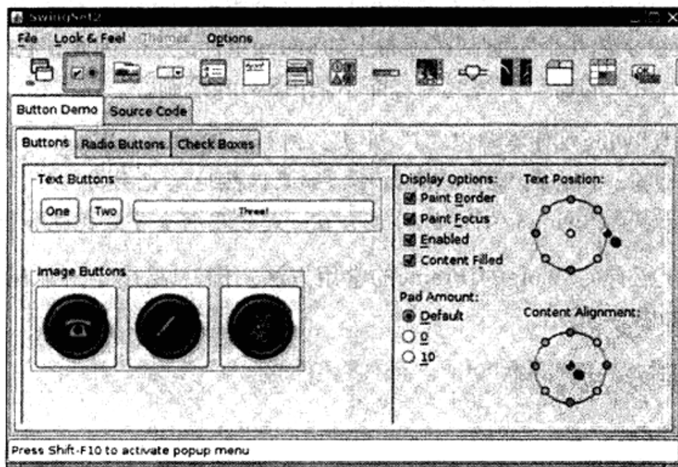
图7-2 Swing的GTK观感
