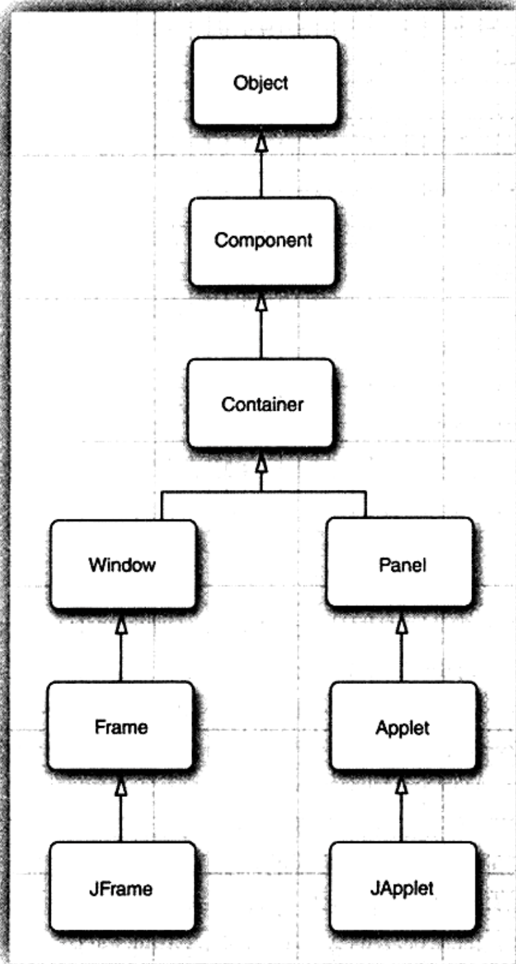
图10-11 Applet继承层次结构
