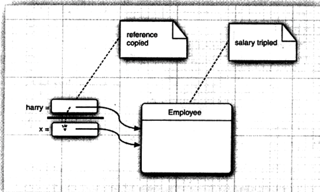
图4-7 对对象参数的修改倍保留了下来
